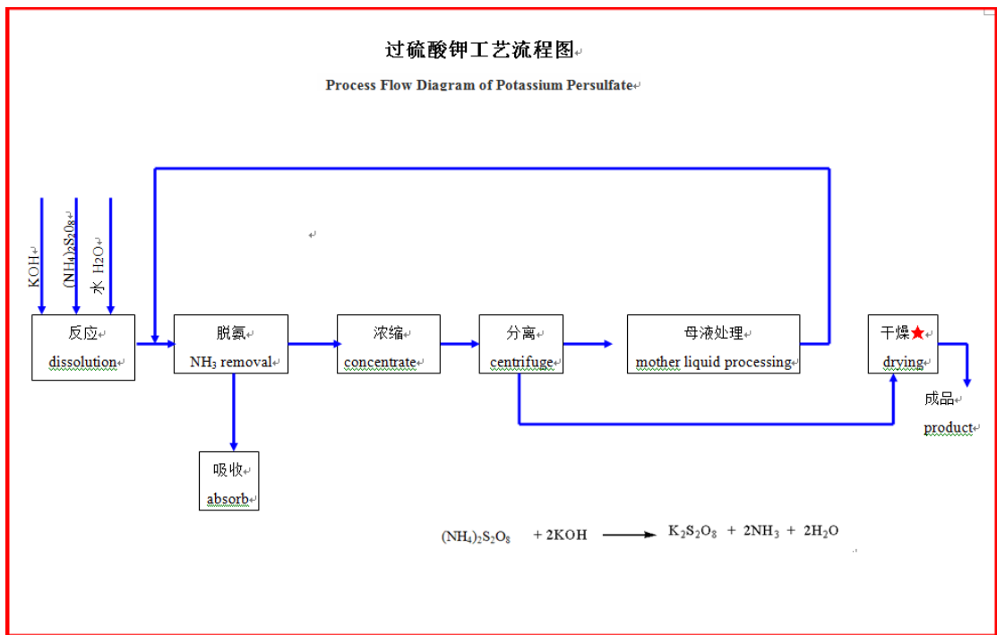
图3 过硫酸钾工艺流程图
