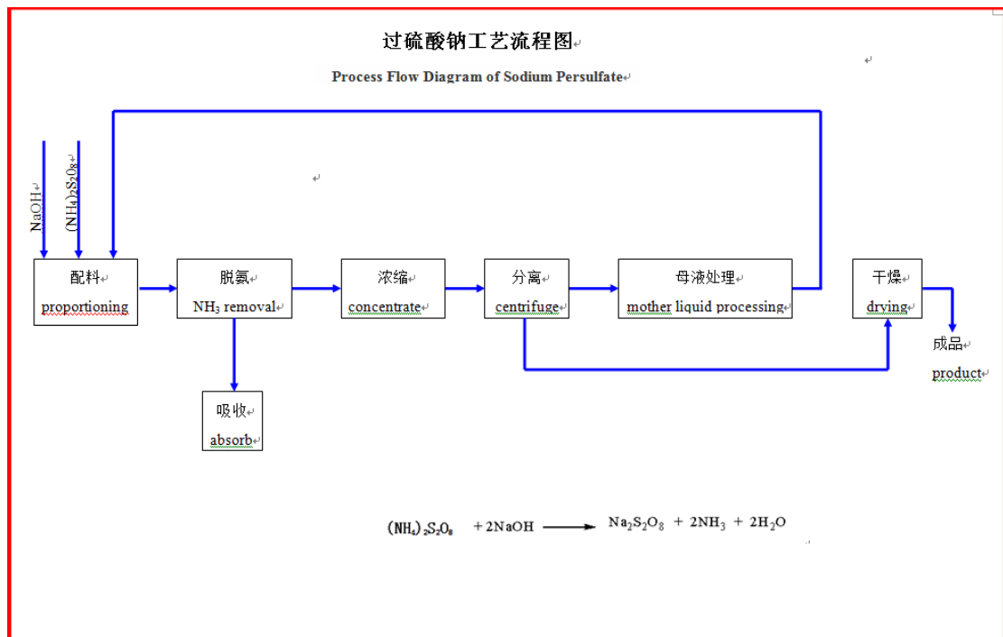
图 2 过硫酸钠工艺流程图
