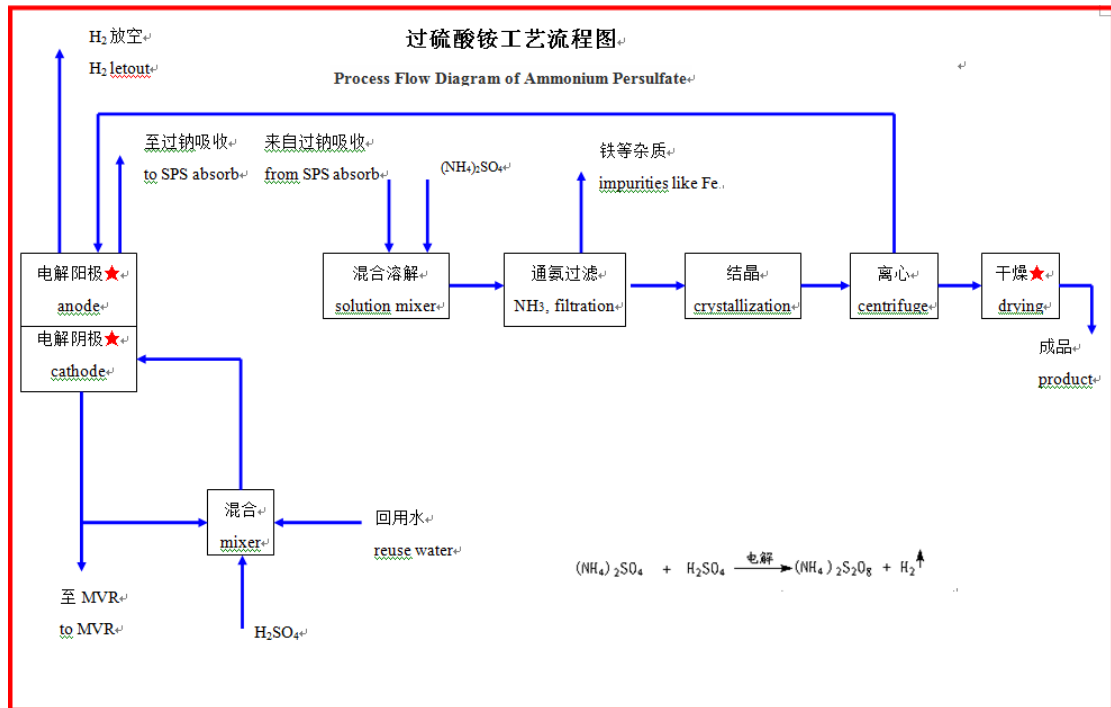
图 1 过硫酸铵工艺流程图
